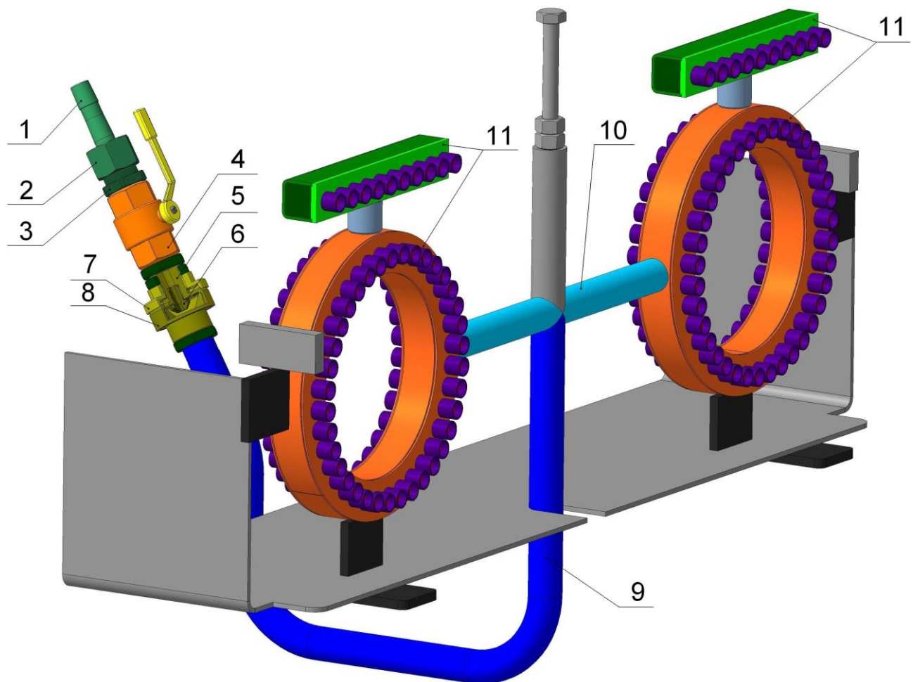
1 – Ниппель; 2 – Гайка; 3 – Штуцер; 4 – Кран; 5 – Трубка; 6 – Инжектор; 7 – Заслонка; 8 – Смеситель; 9 – Трубка; 10 – Трубка; 11 – Мундштук
